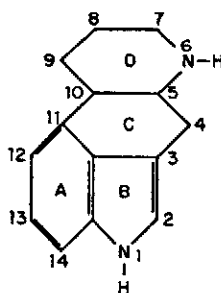
I. Ergoline
